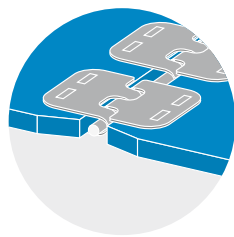
クランプファスナー (メタル)
