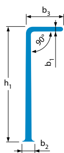
SF-SS (スモールスク ープ棧)
