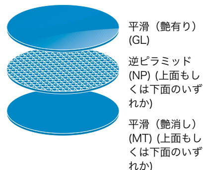
上面コーティング
